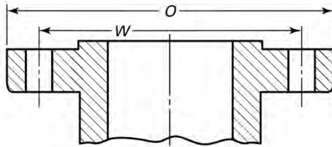
Flange
